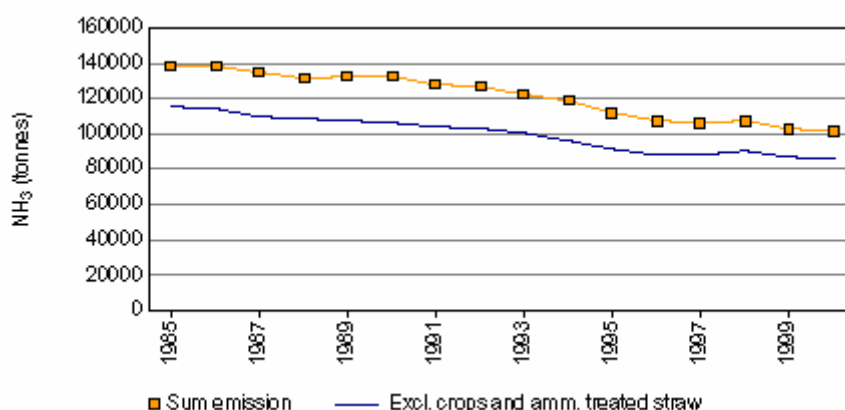
Figur 3.1. Ammoniakemission i Danmark i perioden 1985-2000 (figur fra Illerup et al. 2002)
